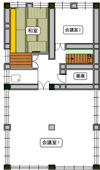
二階平面図
